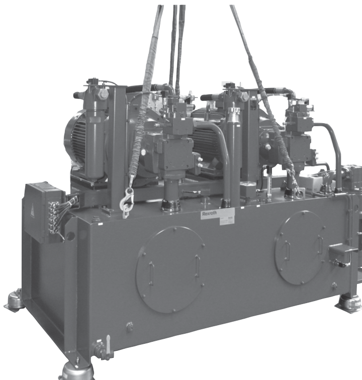
Abb. 5: Verwendung von Hebebändern und Anschlagpunkten
